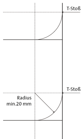
Die sichtbaren Ecken der Abdichtungsbahnen sind abzurunden
